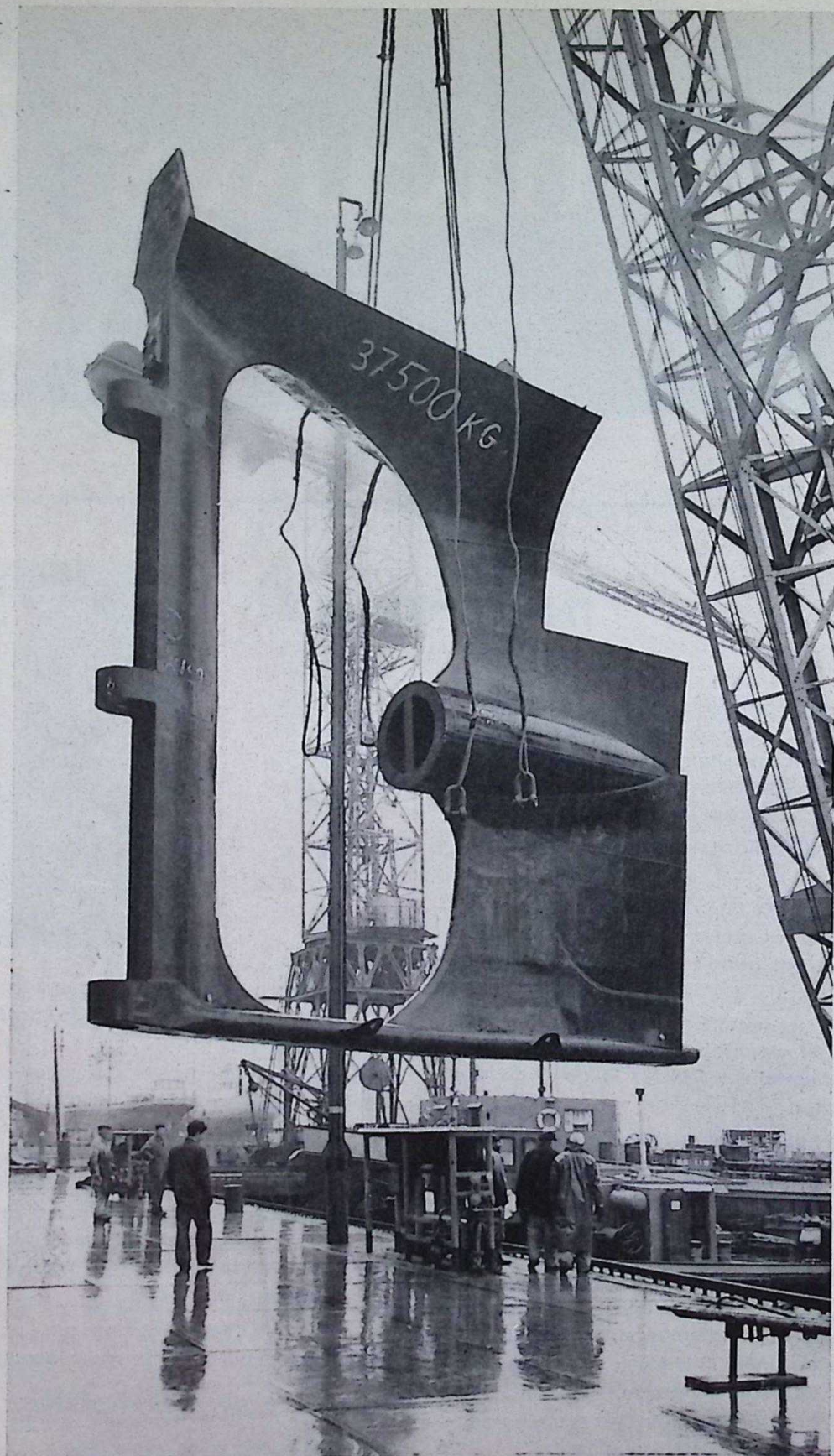
Bovenstaande foto toont weer een staaltje van vakmanschap. Deze achtersteven van 37,5 ton werd bovendien in een recordtijd van ongeveer 2 maanden gebouwd. De achtersteven is bestemd voor een bij de N.V. C. v. d. Giessen en Zn's Scheepswerven in aanbouw zijnd, Engels schip.
