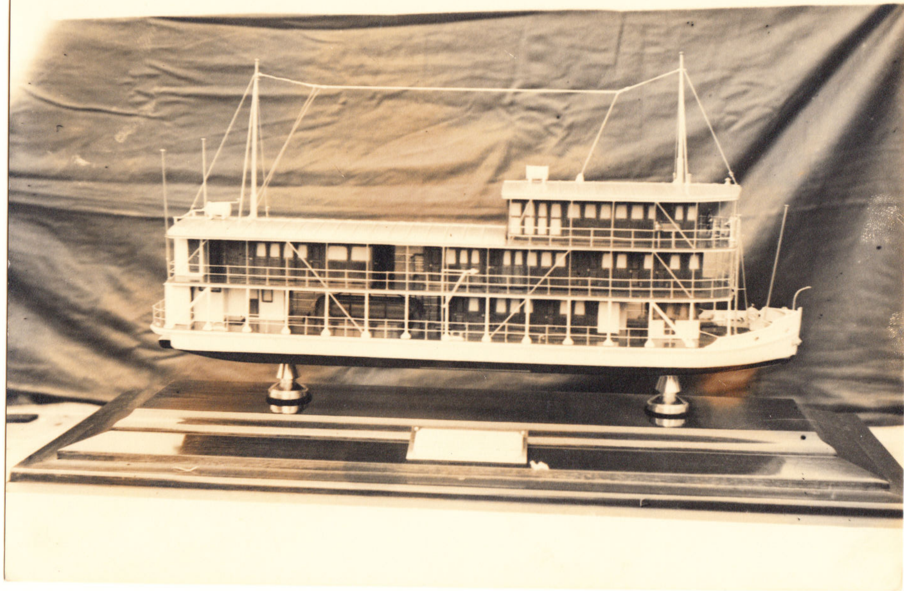
Hogstaatschip voor de Congo 1930 1:50
