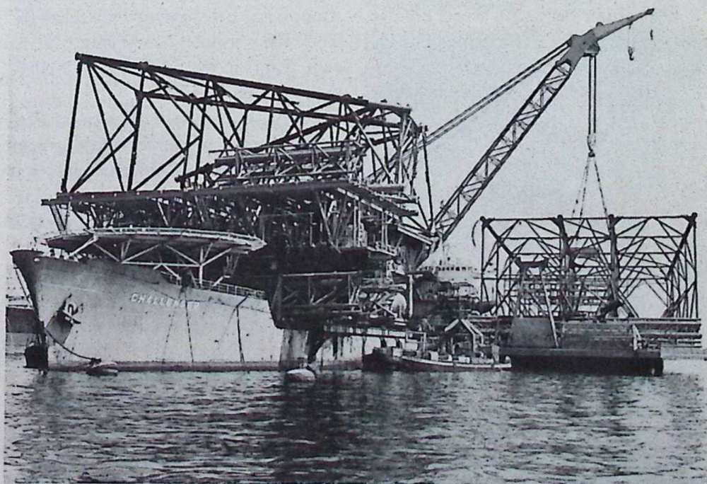
De „Challenger”, door ons omgebouwd tot werkschip, vertrok op 25 augustus met een transport jackets naar de Golf van Suez. Het afgeladen schip bood een onwezenlijke aanblik. Het gebrek aan uitzicht in de stuurhut werd ondervangen door een telefonische verbinding met twee uitkijkposten op het voorschip. U ziet het schip hier tijdens het laden in de Waalhaven op 15 augustus jl. De „Maarten Pieter” ligt langs zij.
