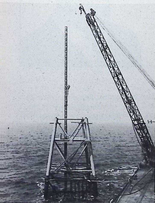
▲ De boorschacht wordt geheid
