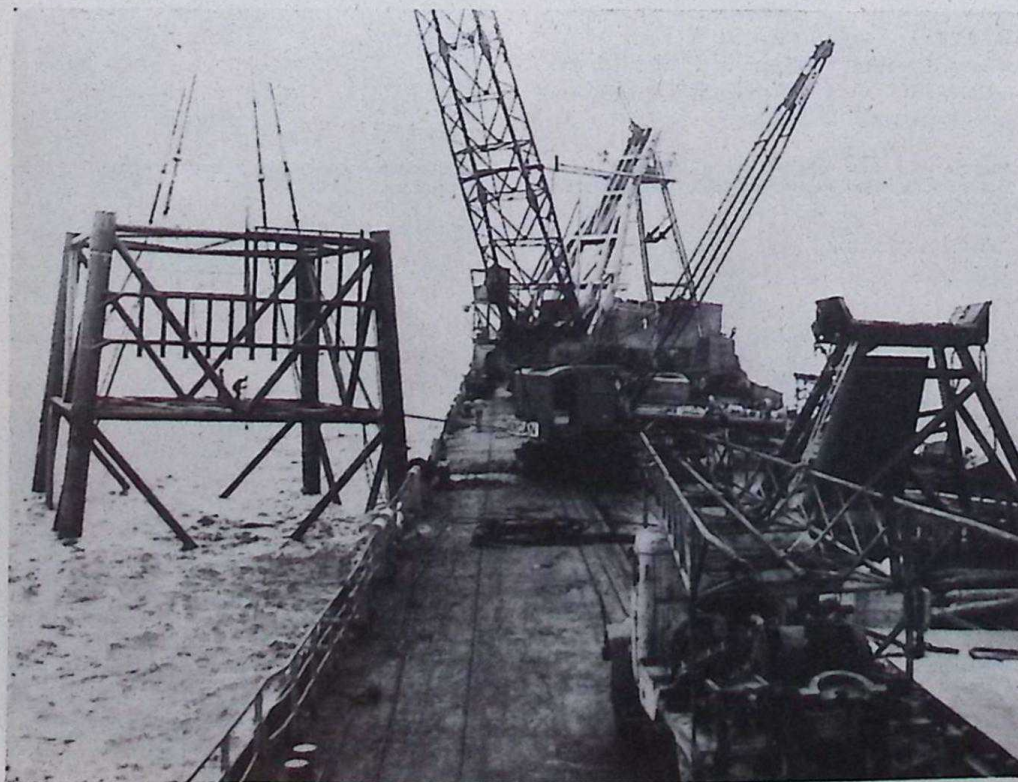
▼ De jacket gaat de zee in
