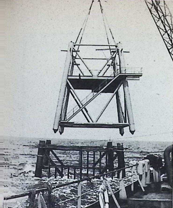
■ sommige jackets gaat er eerst nog een 2e etage op
